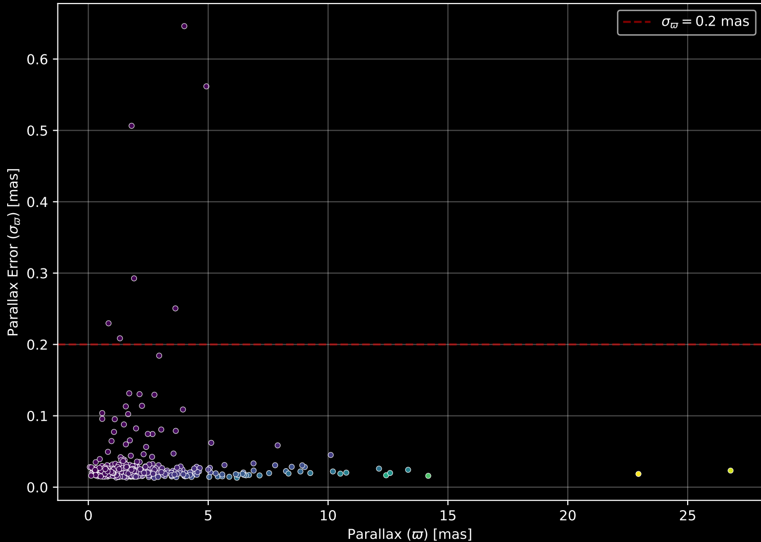
GALAH DR4 Field: [6587] Parallax Quality (n= 471)
