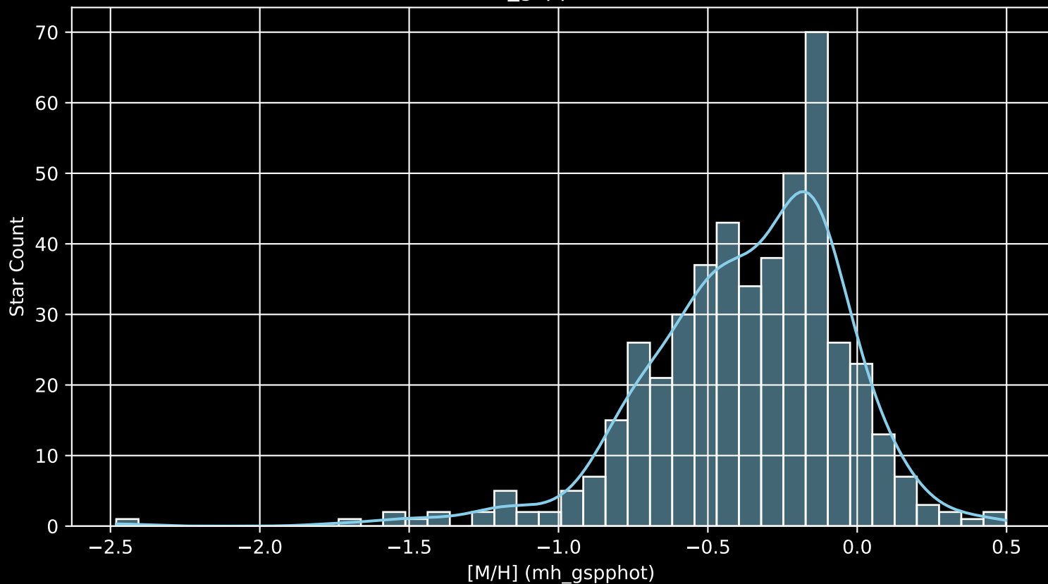
GALAH DR4 Field: [6587] [M/H] (mh_gspphot) (n= 471)
