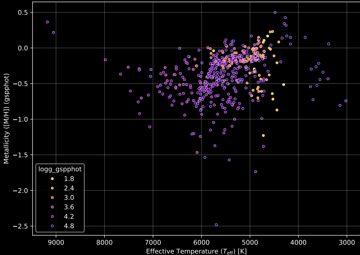
GALAH DR4 Field: [6587] Stellar Population Parameters (n= 471)
